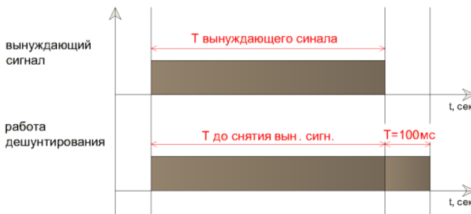
Рисунок 46 – Временная диаграмма работы дешунтирования
