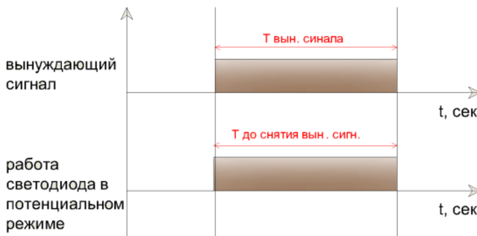
Рисунок 49 – Временная диаграмма работы светодиодов в потенциальном режиме
