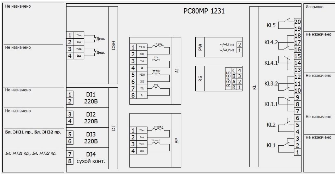
Рисунок 15 – Пример схемы подключения с конфигурацией устройства
