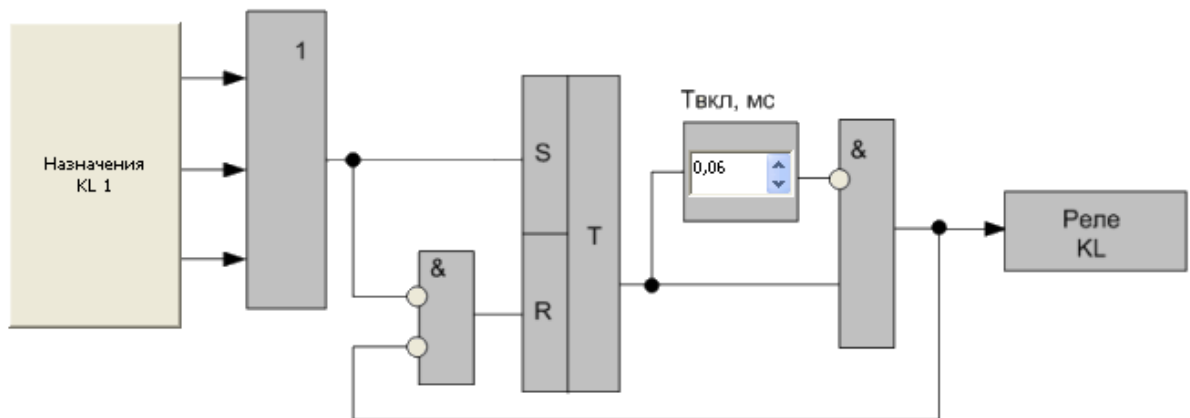
Рисунок 37 - Блок схема алгоритма работы реле KL1 - KL3 в импульсном режиме
