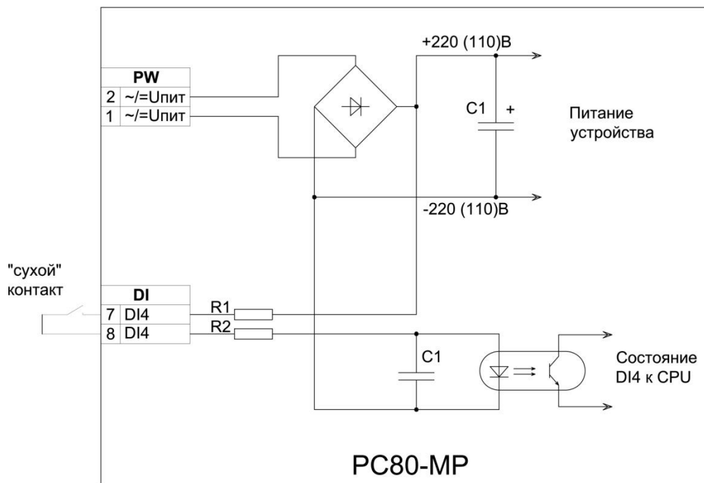
Рисунок 34 – Схема питания дискретного входа DI4
