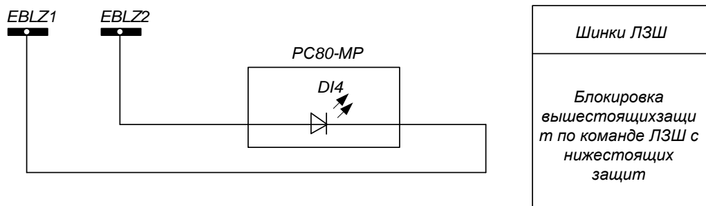
Рисунок 24 – Схема организации блокировки быстродействующих ступеней последующих защит (выключатель ввода, секционный выключатель) через DI4
