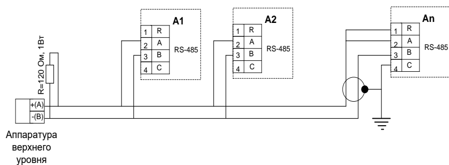
Рисунок 52 – Организация локальной сети
