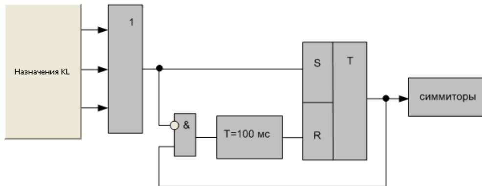
Рисунок 45 - Блок схема алгоритма работы дешунтирования
