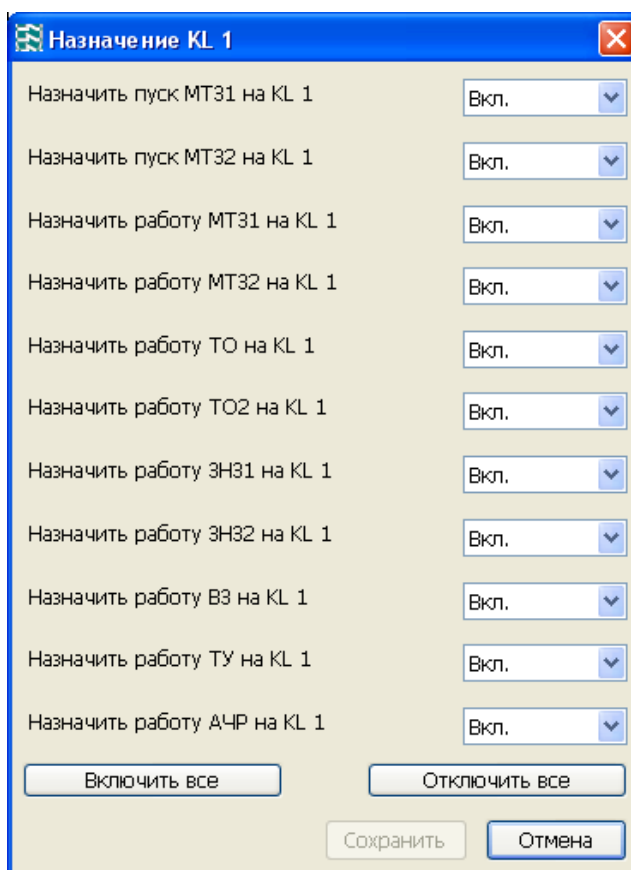
Рисунок 35 – Варианты назначений на выходные реле KL1 – KL3 , работающих на отключение
