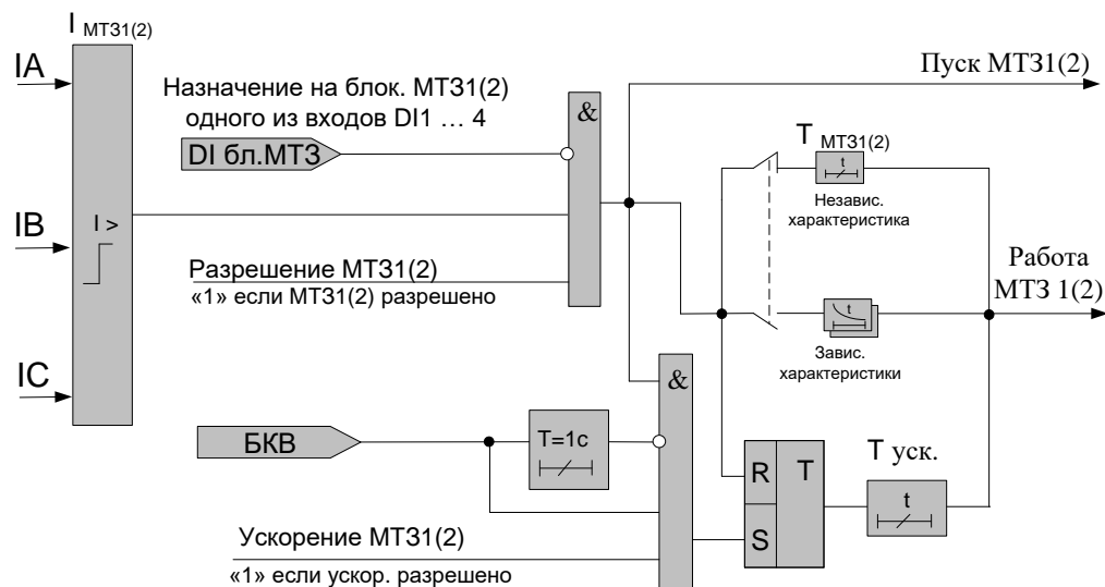
Рисунок 17 – Функциональная схема МТЗ1(2)
