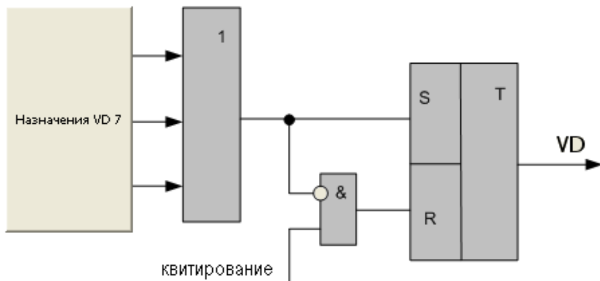
Рисунок 50 – Блок схема алгоритма работы светодиода в режиме с фиксацией
