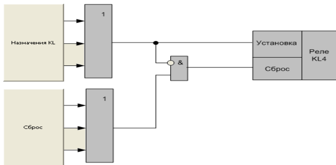
Рисунок 41 – Блок схема алгоритма работы реле KL4
