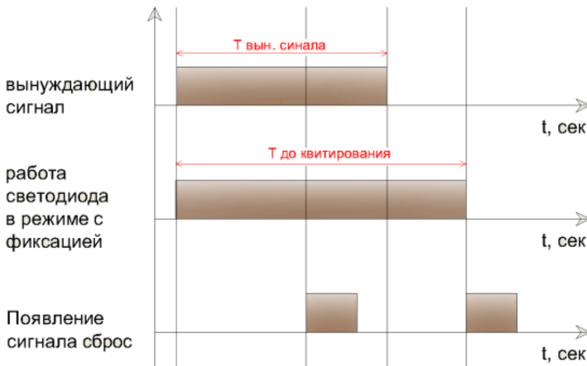
Рисунок 51 – Временная диаграмма работы светодиодов в режиме с фиксацией
