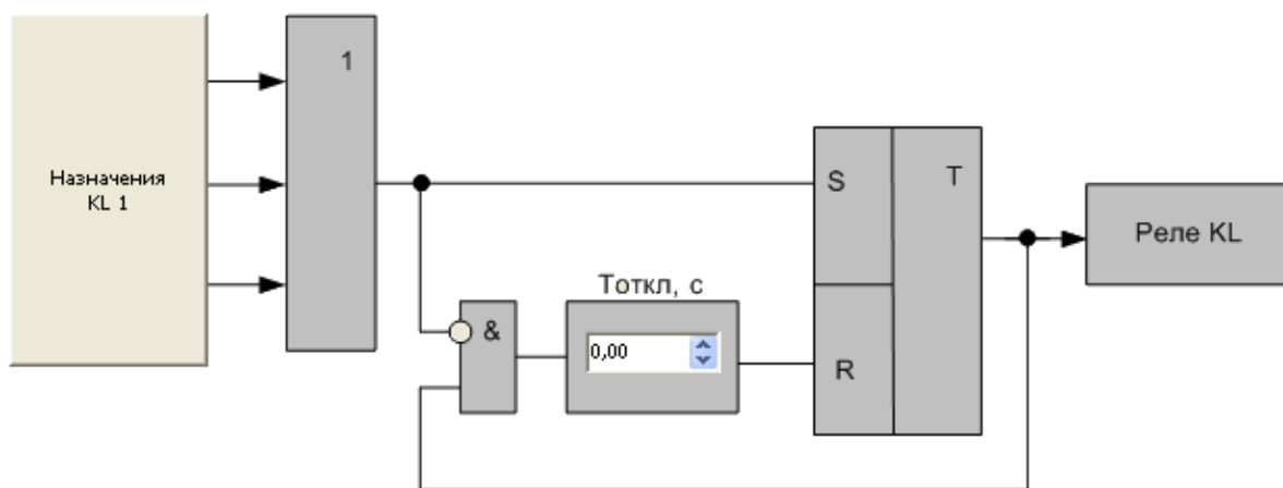
Рисунок 39 – Блок схема алгоритма работы реле KL1 - KL3 в потенциальном режиме
