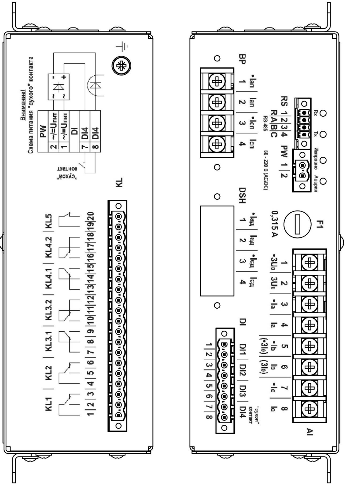
Рисунок Б.4 – Схема расположения выводов для подключения к устройству РС80-МР исполнений: РС80-МР-хх2х
