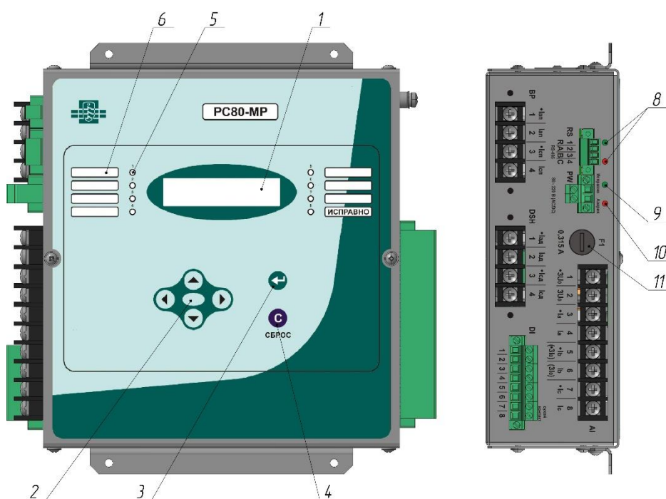
Рисунок 16 – Расположение элементов управления и индикации устройства
