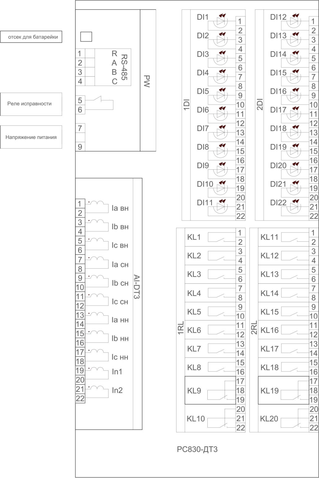
Рисунок Б.2 – Схема подключения устройства PC830-DT3 (исполнений XX22XXXXXX)
