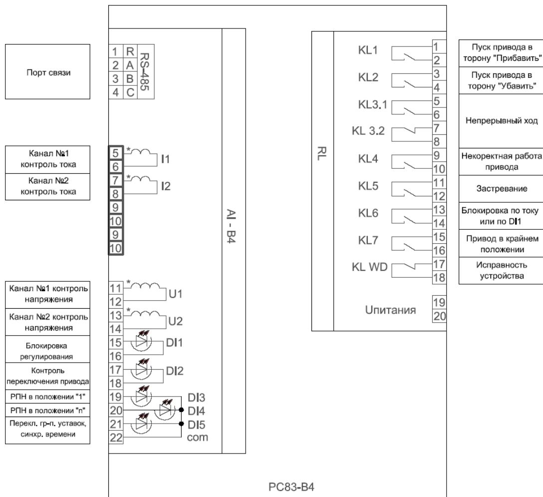
Рисунок 12 – Схема подключения PC83-B4 без модуля датчиков положения РПН
