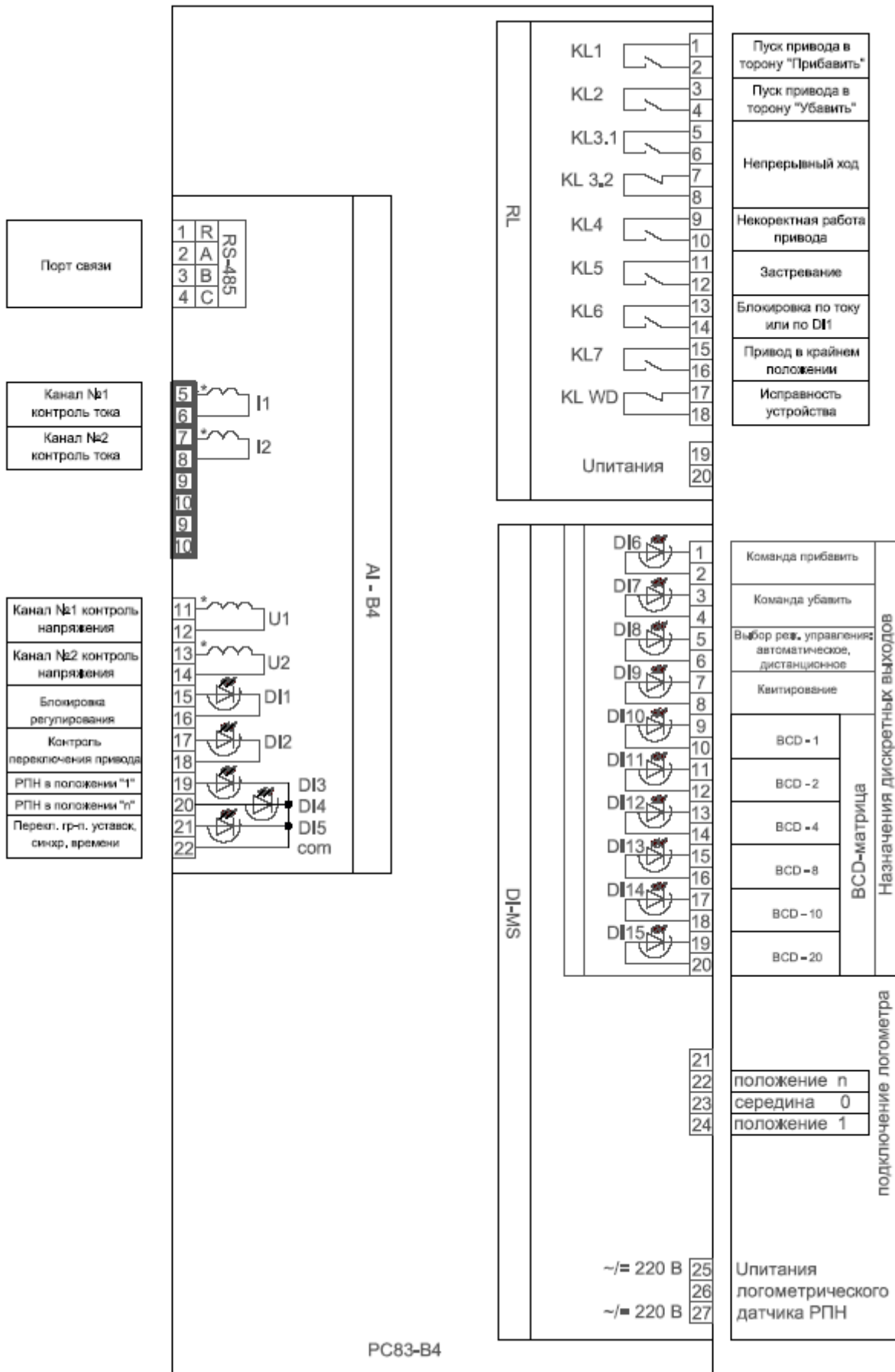
Рисунок 13 – Схема подключения РС83-В4 с модулем датчиков положения РПН
