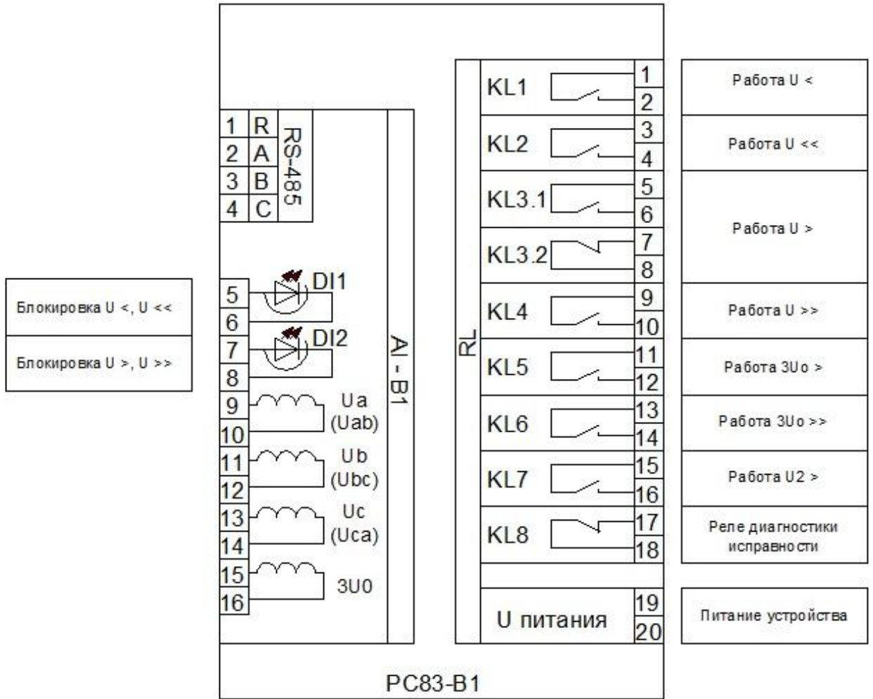
Рисунок 4 – Схема подключения PC83-B1
