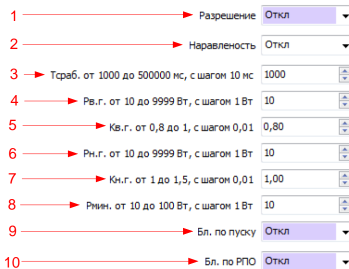
Рисунок 23 – Окно настроек КАМ в программе «BURZA»
