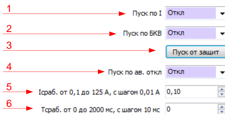
Рисунок 74 – Окно уставок УРОВ в программе «BURZA»
