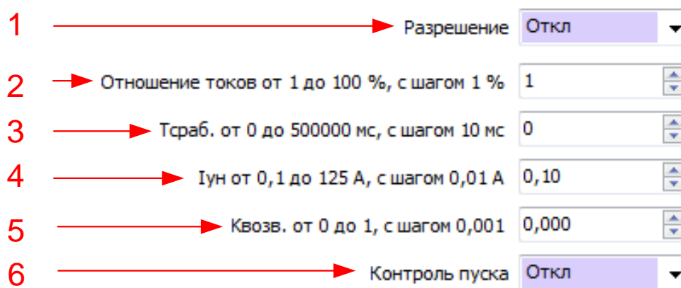
Рисунок 48 – Окно настроек ЗНР в программе «BURZA»
