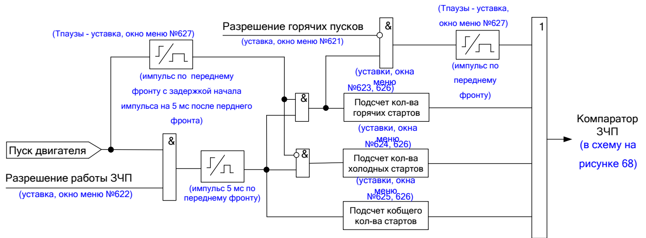
Рисунок 70 – Функциональная схема логики компаратора ЗЧП
