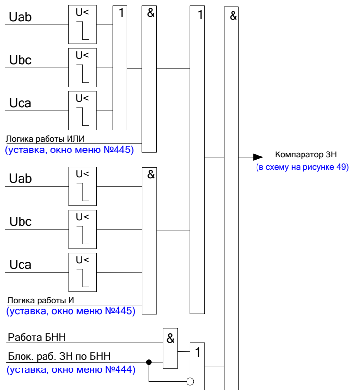
Рисунок 52 – Функциональная схема логики компаратора ЗН при работе в режиме ЗМН по линейным напряжениям
