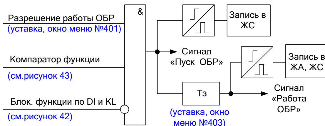
Рисунок 41 – Фрагмент функциональной схемы логики ОБР
