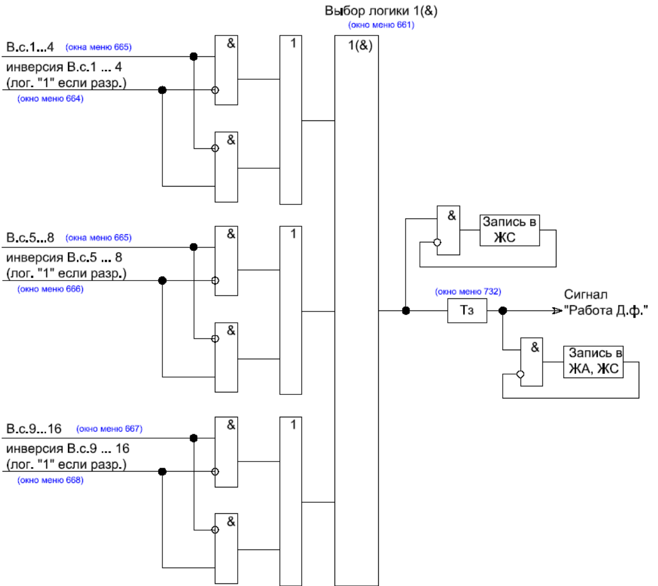
Рисунок 31 – Фрагмент функциональной схемы логики Дф
