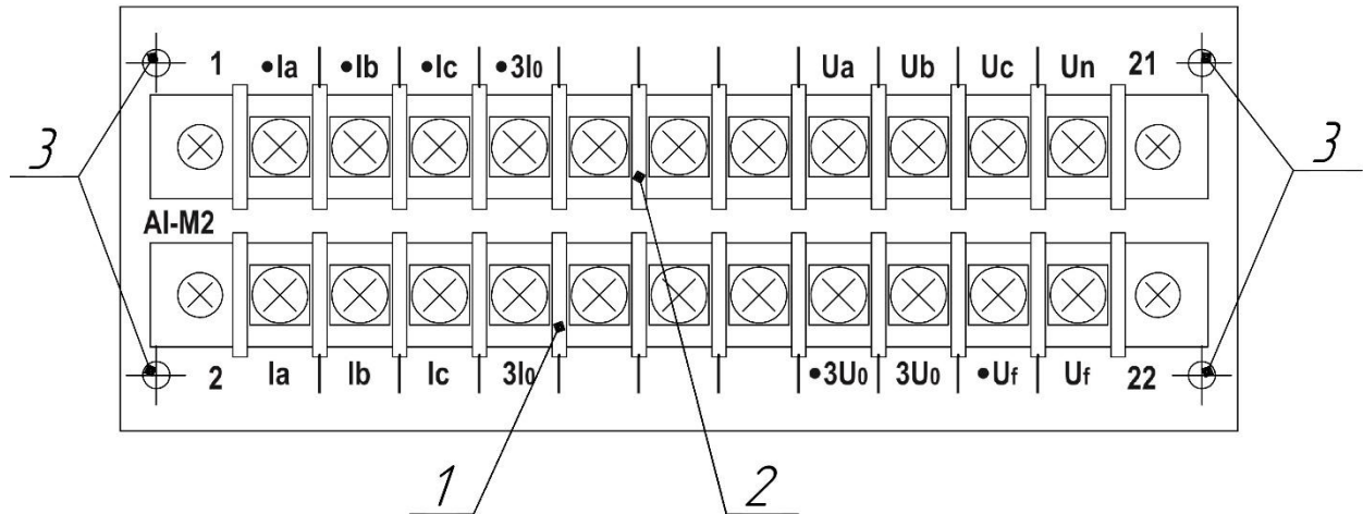
Рисунок 11 – Модуль AI-M2 (вид со стороны разъемов для внешних подключений) и его маркировка
