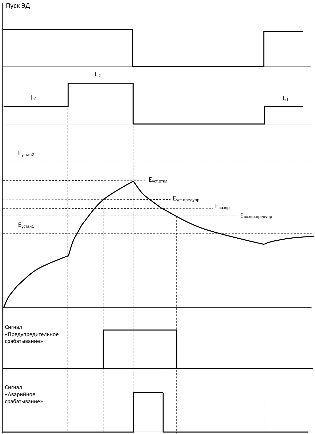
Рисунок 76 - Диаграммы работы ТЗ
