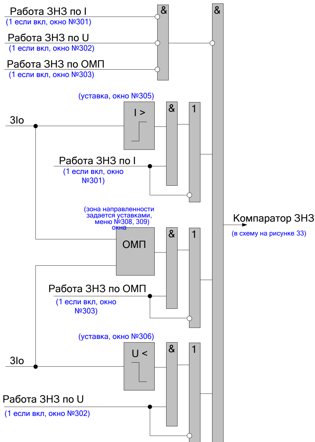
Рисунок 35 – Функциональная схема логики компаратора ЗНЗ
