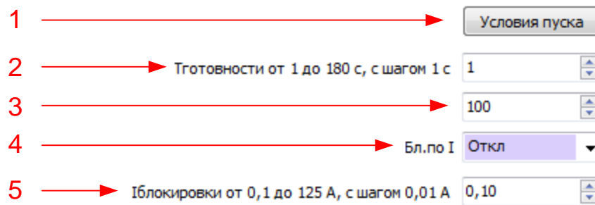
Рисунок 80 – Окно уставок АПВ в программе «BURZA»
