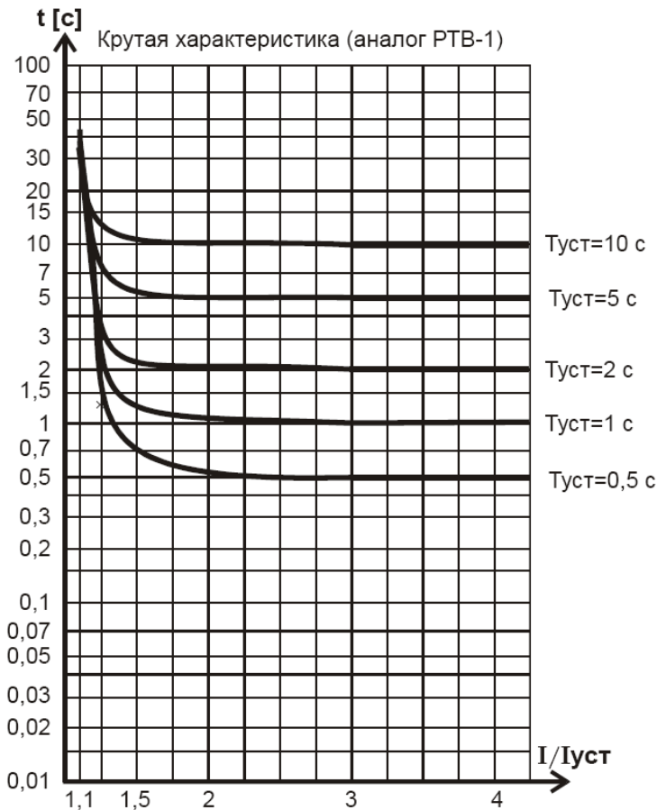
Крутая характеристика (аналог РТВ-1)
