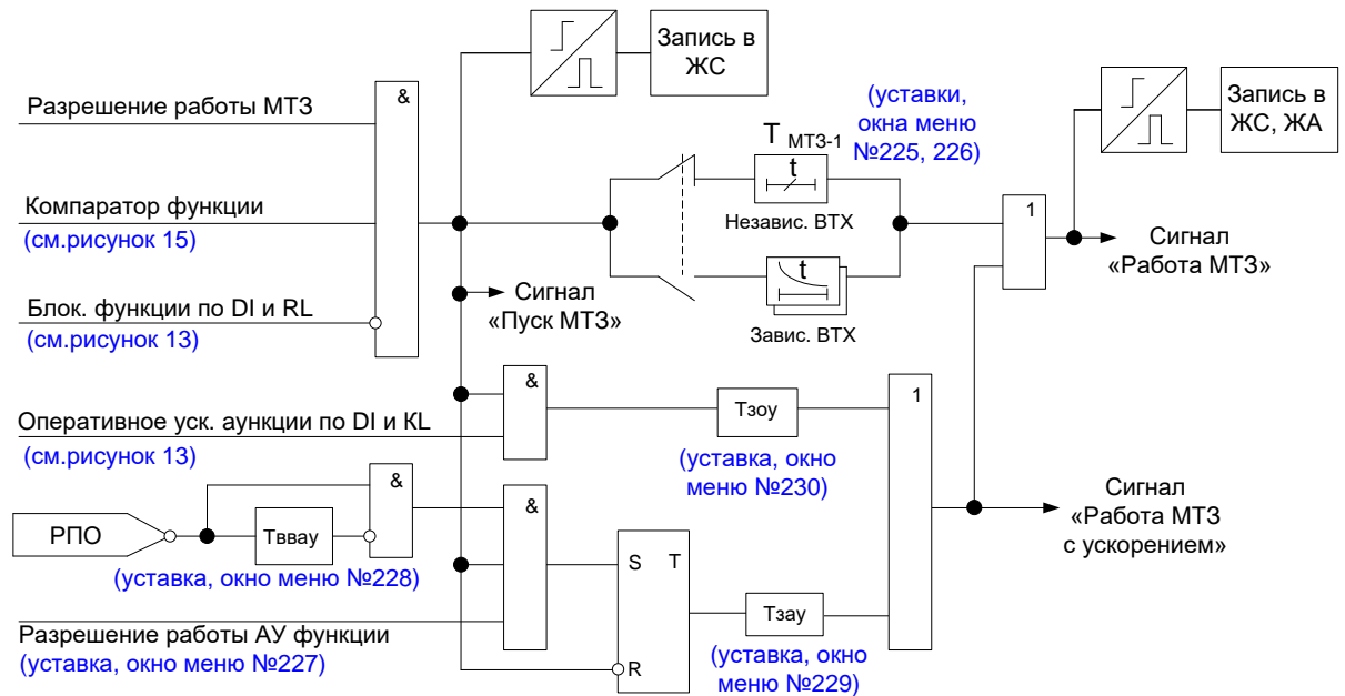
Рисунок 12 – Фрагмент функциональной схемы логики МТЗ
