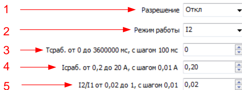
Рисунок 44 – Окно настроек ОБР в программе «BURZA»
