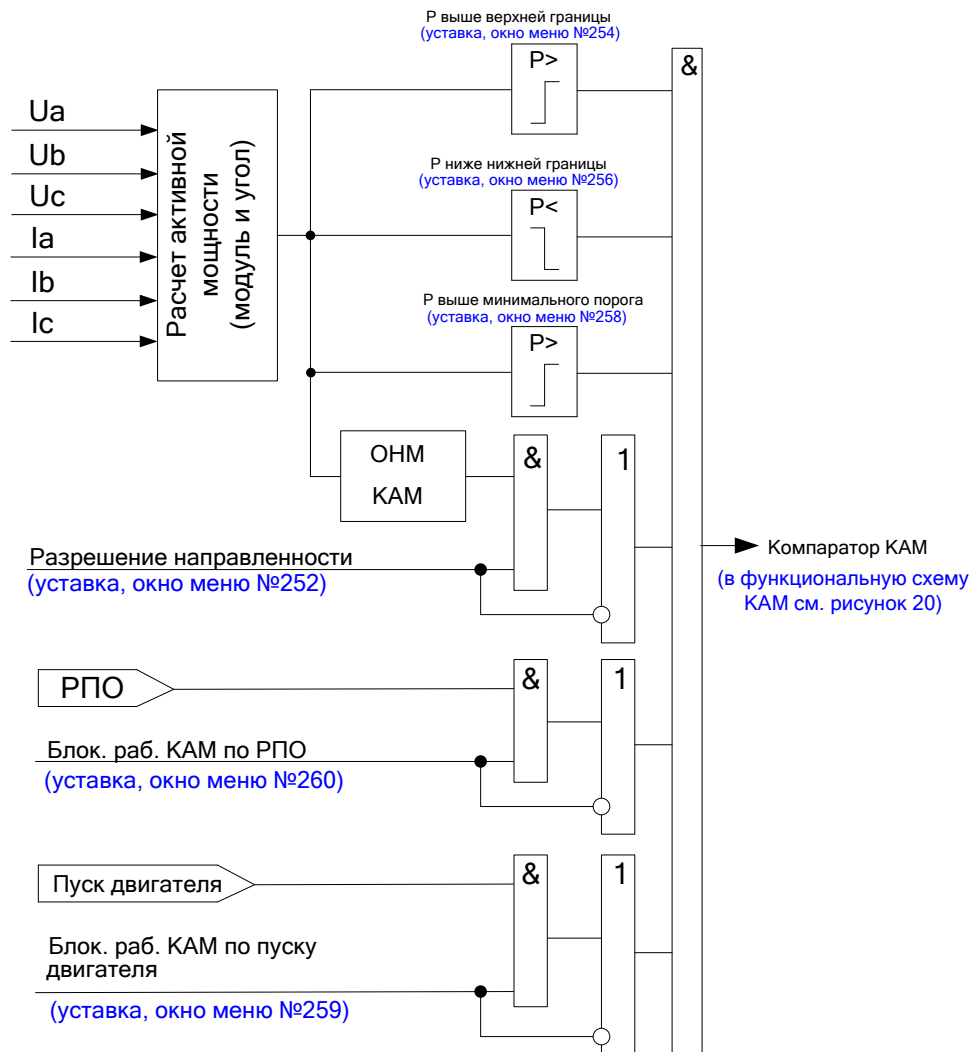
Рисунок 22 – Функциональная схема логики компаратора КАМ
