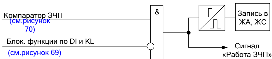
Рисунок 68 – Фрагмент функциональной схемы логики ЗЧП
