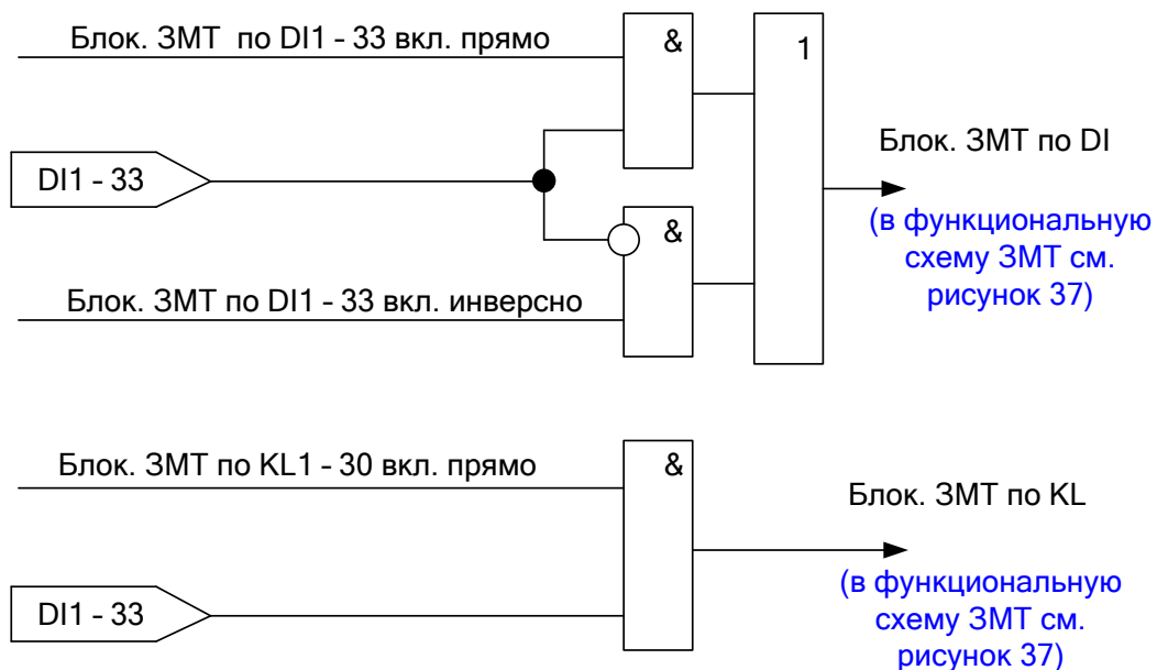
Рисунок 38 – Алгоритм формирования сигналов блокировки ЗМТ по дискретным входам и логическим выходам реле
