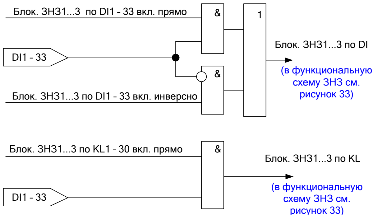
Рисунок 34 – Алгоритм формирования сигналов блокировки ЗНЗ по дискретным входам и логическим выходам реле
