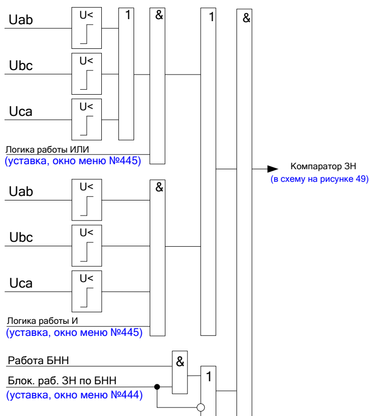
Рисунок 53 – Функциональная схема логики компаратора ЗН при работе в режиме ЗПН по линейным напряжениям
