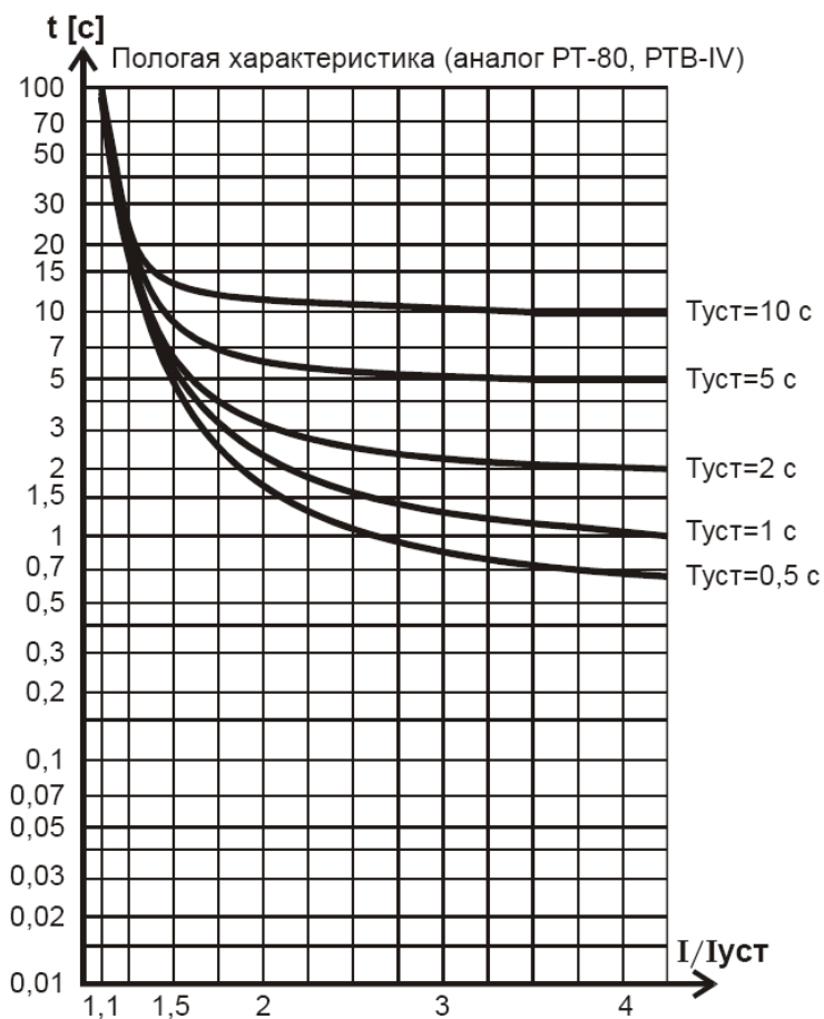
Пологая характеристика (типа реле РТ-80, РТВ-IV)
