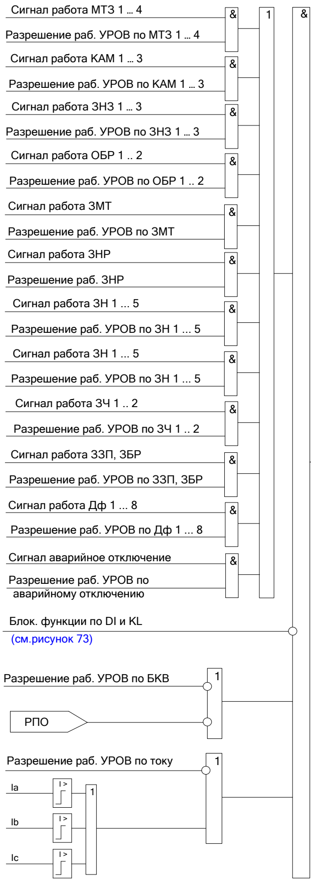
Рисунок 72 – Блок схема алгоритма УРОВ
