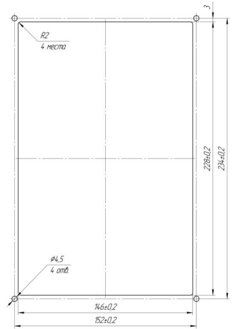
Отверстия для внутреннего монтажа устройства (вырез в панели)
