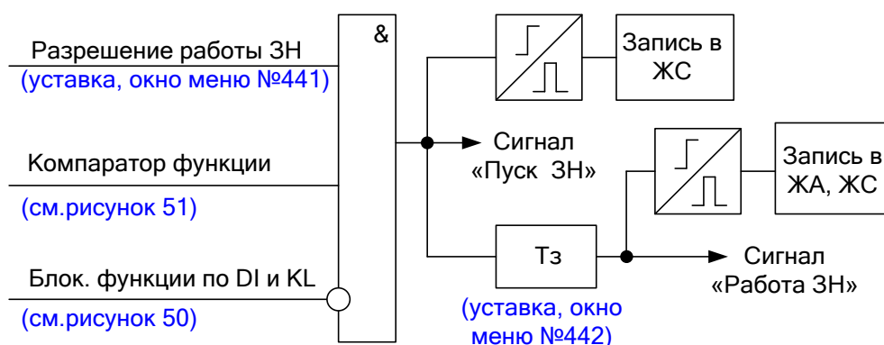
Рисунок 49 – Фрагмент функциональной схемы логики ЗН
