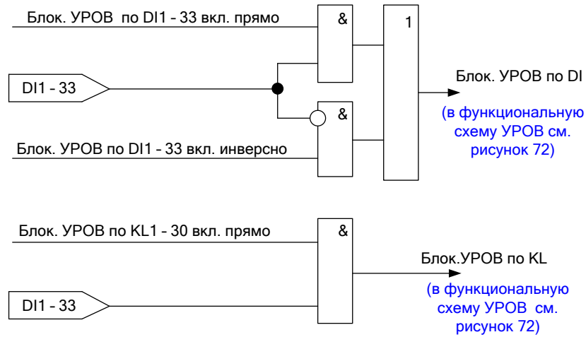
Рисунок 73 – Алгоритм формирования сигналов блокировки УРОВ по дискретным входам и логическим выходам реле
