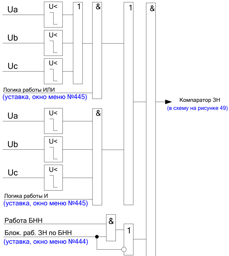
Рисунок 51 – Функциональная схема логики компаратора ЗН при работе в режиме ЗМН по фазным напряжениям
