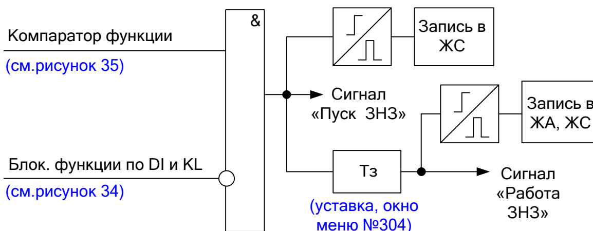
Рисунок 33 – Фрагмент функциональной схемы логики ЗНЗ
