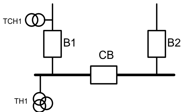
Рисунок 85 – Выявление неисправности цепей напряжения с использованием информации от второго трансформатора (ТСН или ТН)
