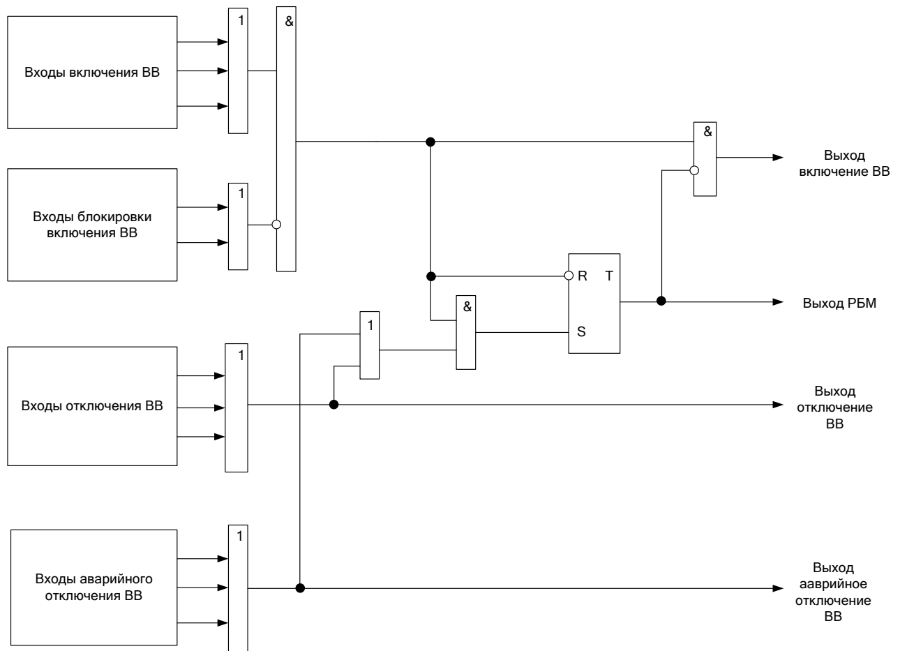
Рисунок 82 – Блок схема алгоритма работы АУВ
