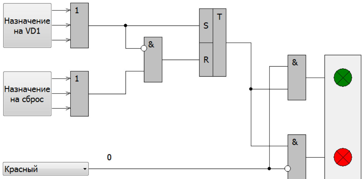
Рисунок 97 – Алгоритм работы светодиодов в режиме с фиксацией
