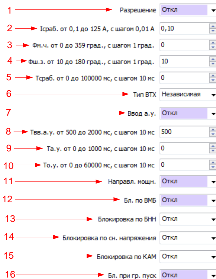
Рисунок 19 – Окно настроек МТЗ в программе «BURZA»
