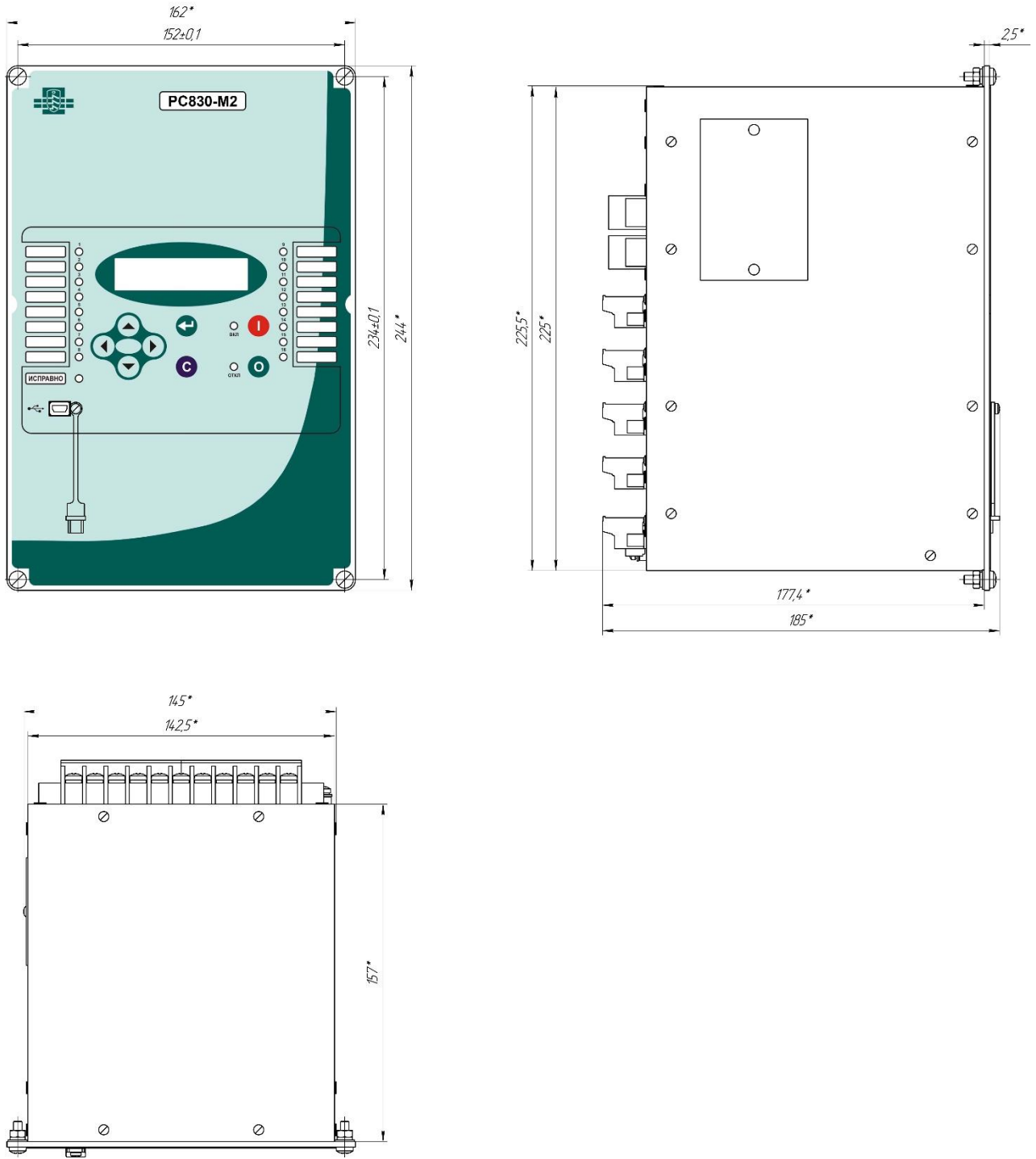
Рисунок Б.1 – Габаритные и присоединительные размеры устройства PC830-M2
