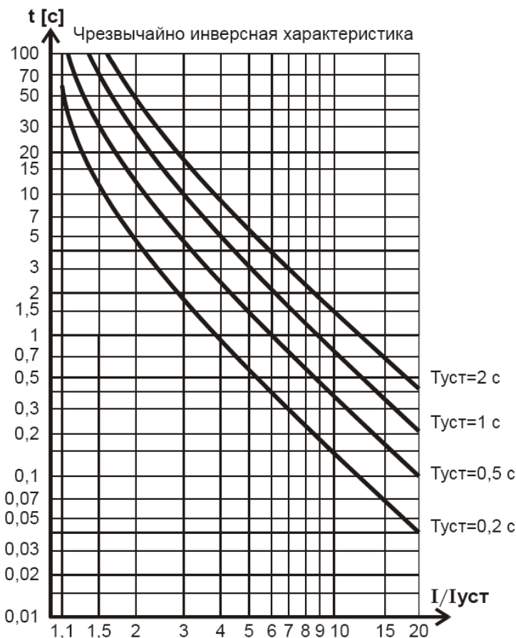
Чрезвычайно инверсная характеристика по МЭК 255-4
