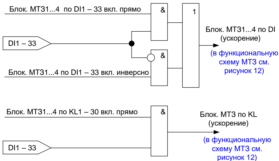
Рисунок 13 – Алгоритм формирования сигналов блокировки (ускорения) МТЗ по дискретным входам и логическим выходам реле Конфигурация МТЗ представлена в таблице 9.
