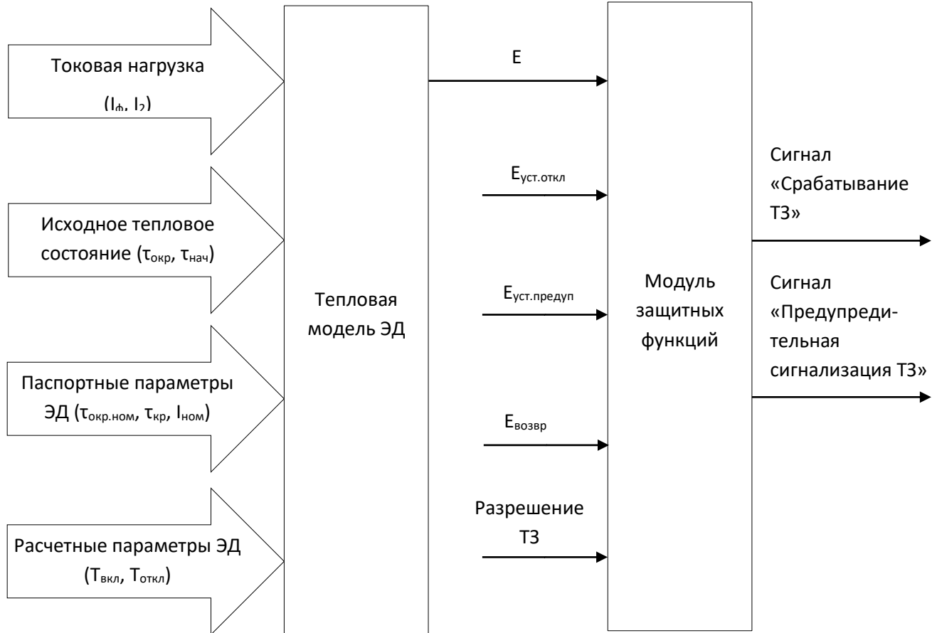
Рисунок 75 - Структура ТЗ
