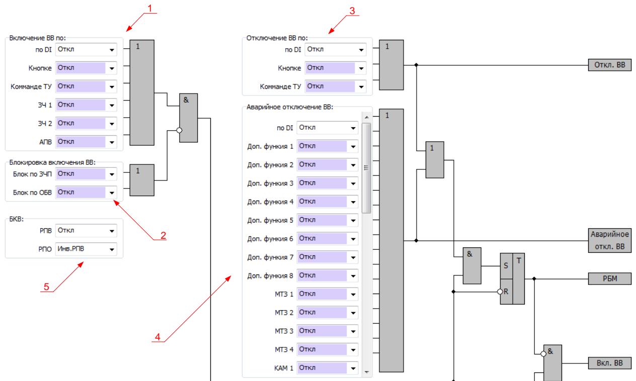
Рисунок 83 – Окно уставок АУВ в программе «BURZA»
