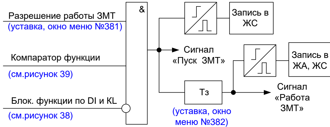
Рисунок 37 – Фрагмент функциональной схемы логики ЗМТ
